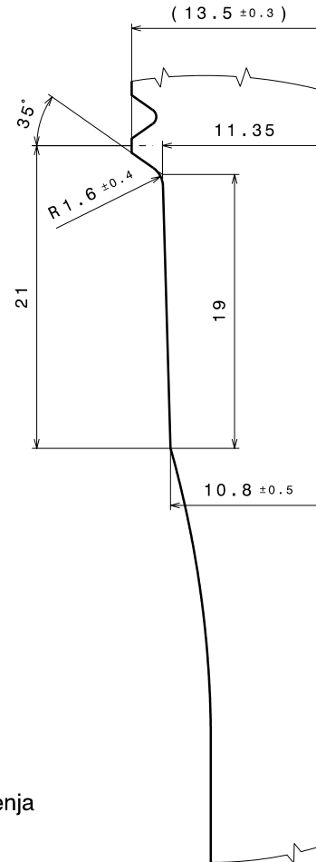
detalj E
