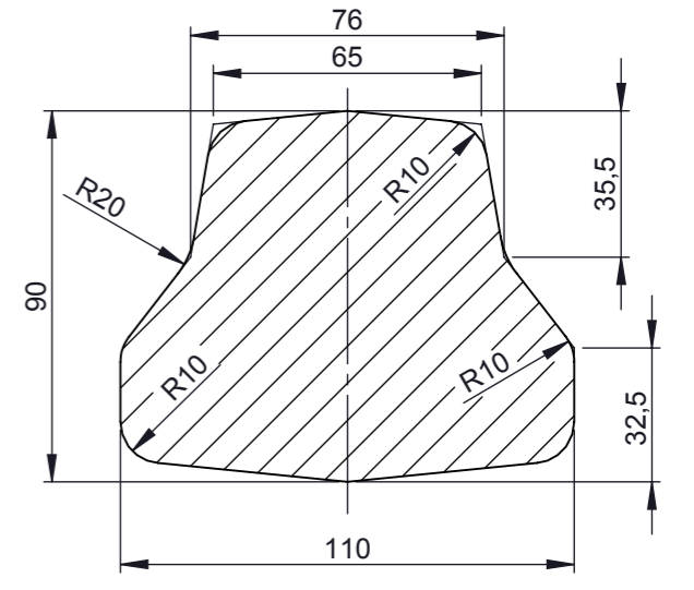
PRESEK A-A Razmera 1 : 2
