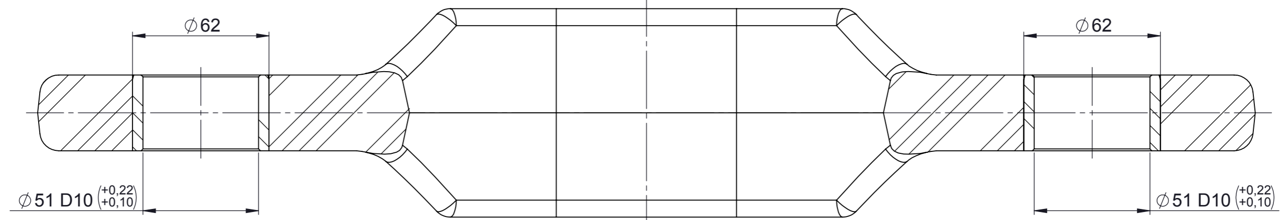
PRESEK A-A RAZMERA 1 : 2
