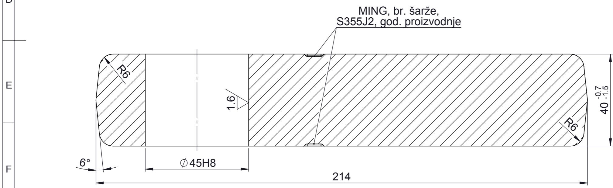
PRESEK A-A
