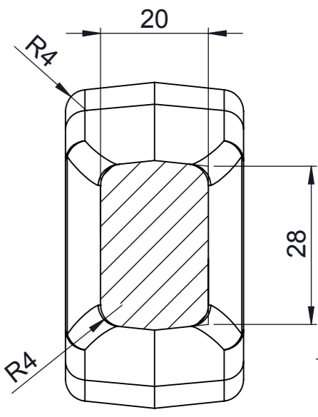
PRESEK B-B
