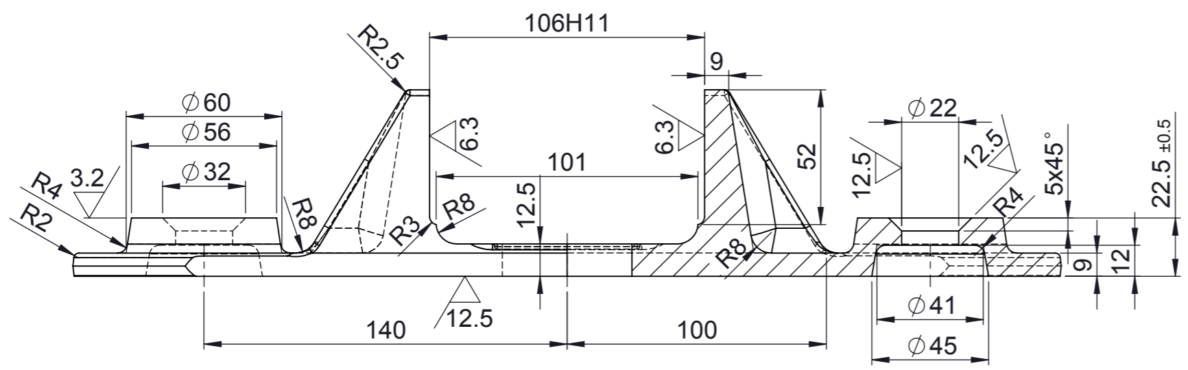
PRESEK A-A
