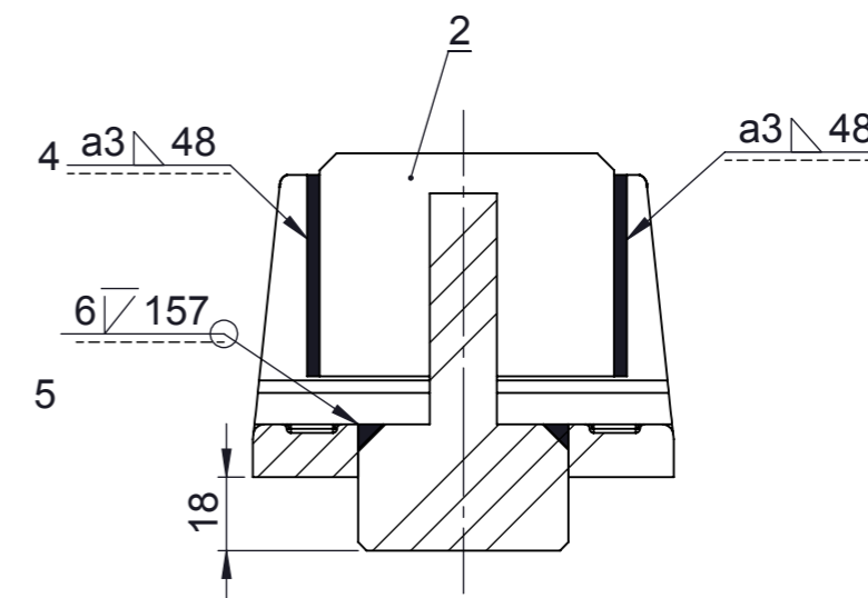
PRESEK A-A
